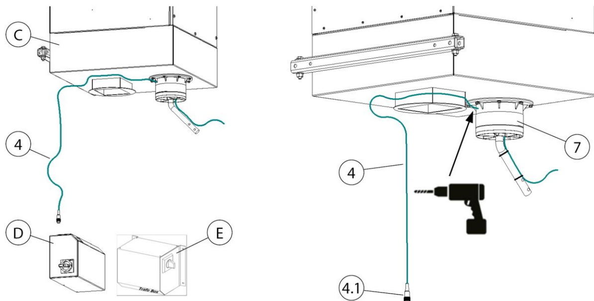
Fig. 19 : Pose des câbles – appareil stationnaire
