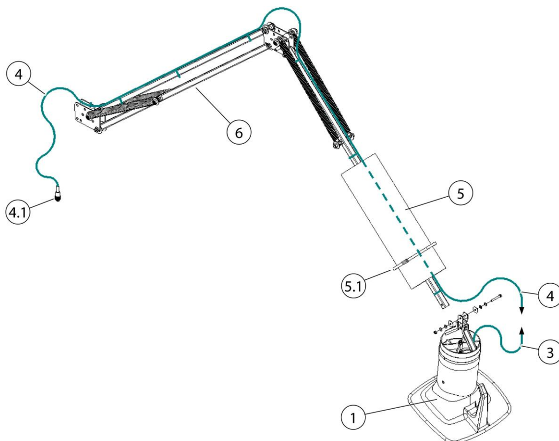
Fig. 18 : Pose des câbles - bras d'aspiration 2-4 mètres
