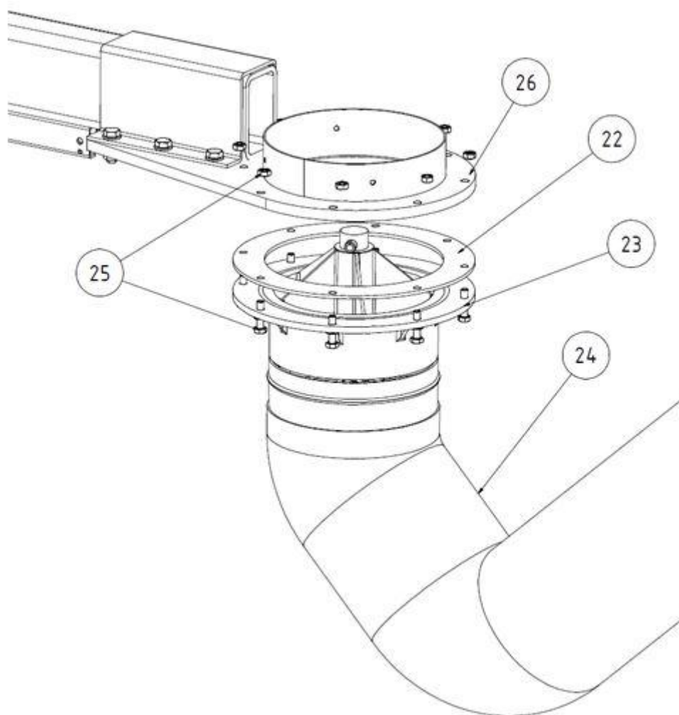
Fig. 12 : Bras d'aspiration sur potence
