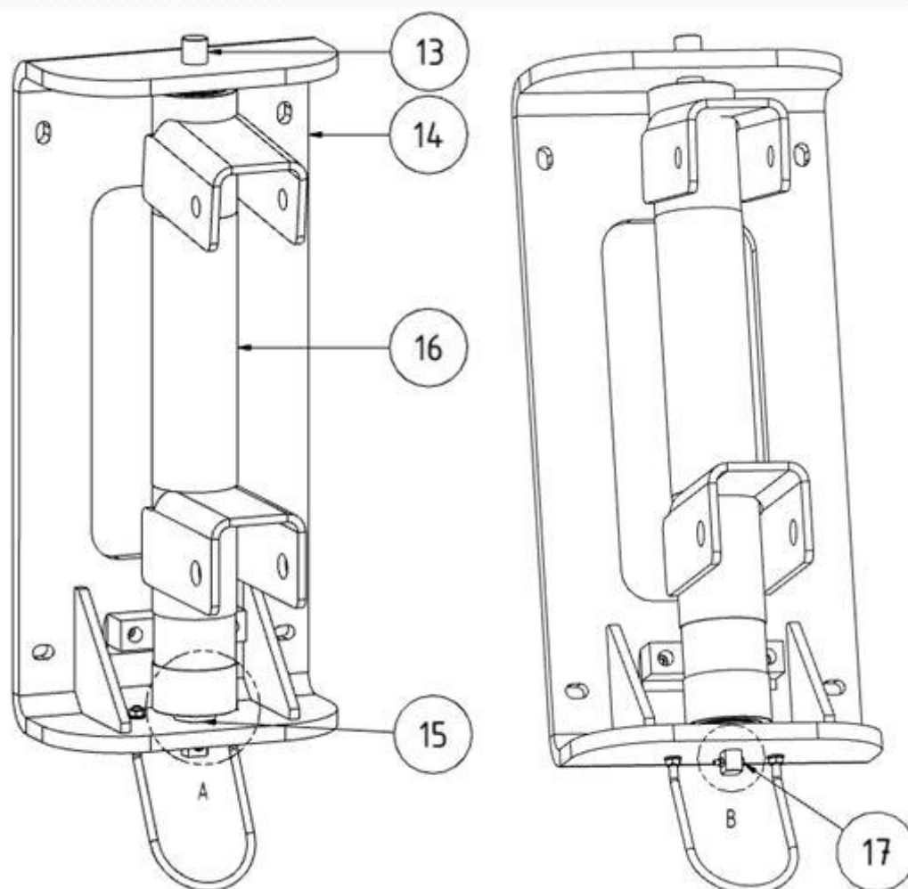
Fig. 6 : Support de la potence
