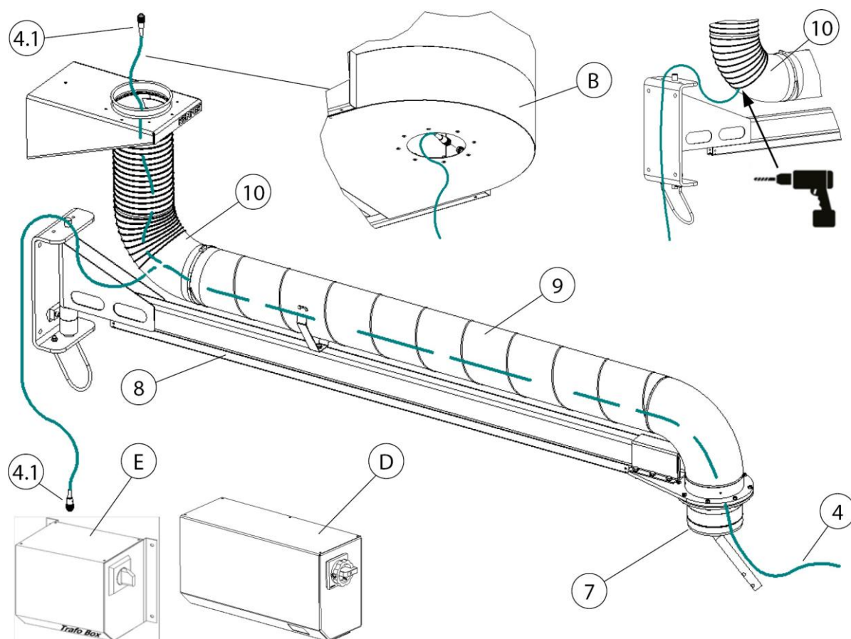
Fig. 17 : Pose des câbles – bras d'aspiration avec potence
